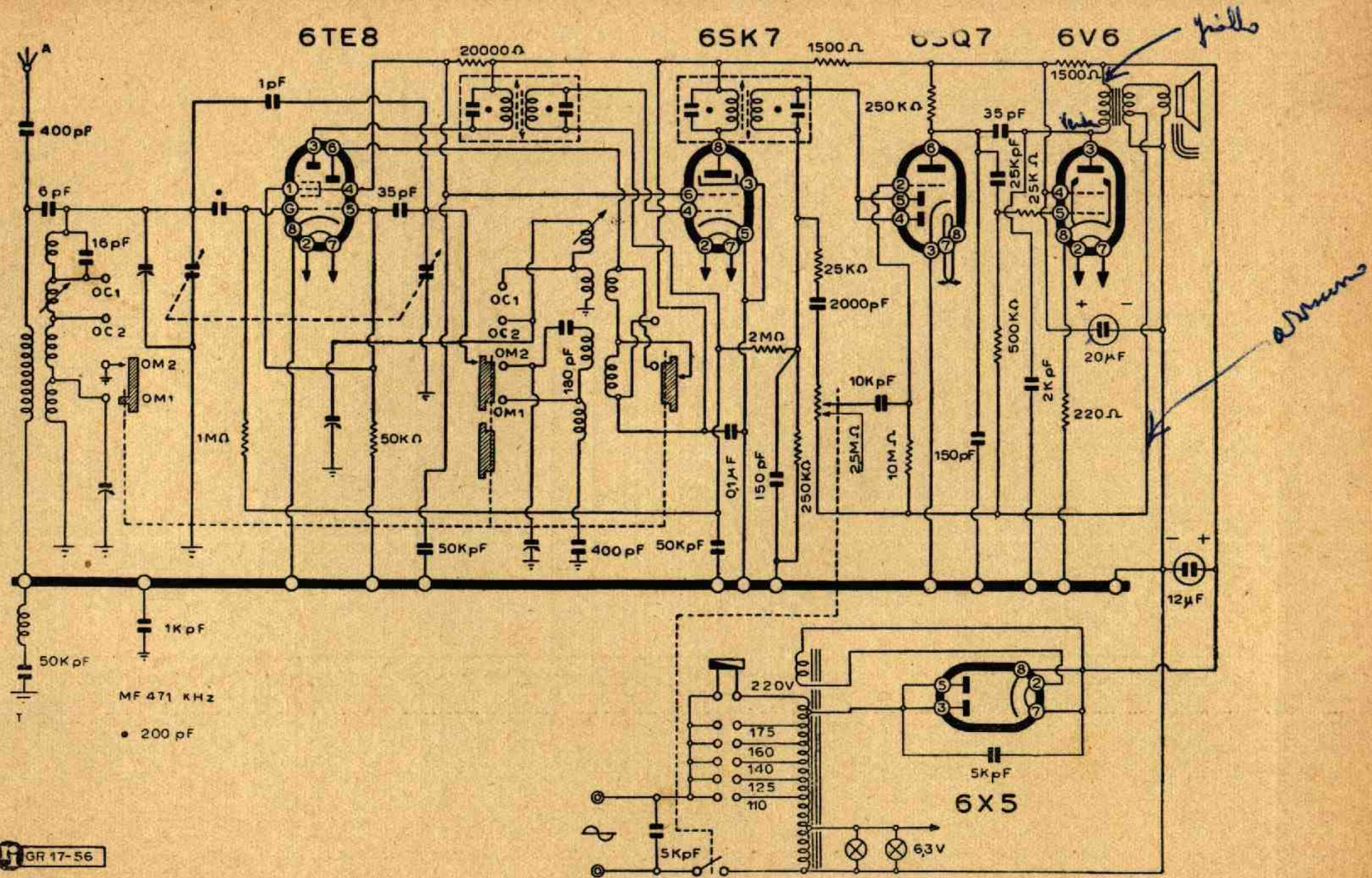
Lo schema elettrico dell' S 23
